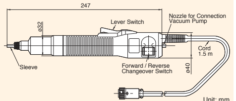
DLV7325/7335/7319/7329/7339
