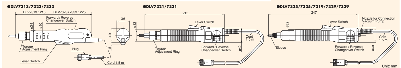
DLV7325/7335/7319/7329/7339
