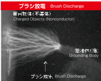
山陽瑞樹 フレキシブルコンテナに関連した労働災害と規格の動向 69P 図 2(b) ブラシ放電「労働安全衛生研究」Vol.7, No.2, pp.67-76 (2014) より Written by Mizuki Yamaguma, Title: Labor Accidents and Standards in Association with Flexible Intermediate Bulk Containers (FIBC), From Journal of Occupational Health and Safety, Vol 7, No.2, pp.67-76 (2014)
